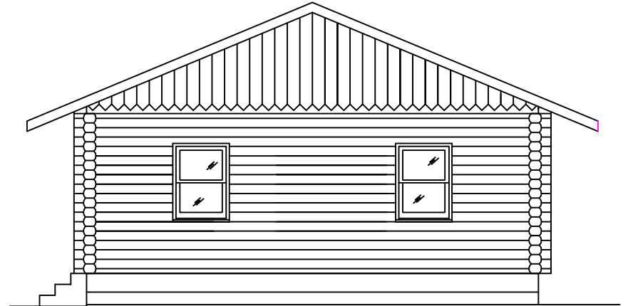
RIGHT ELEVATION
