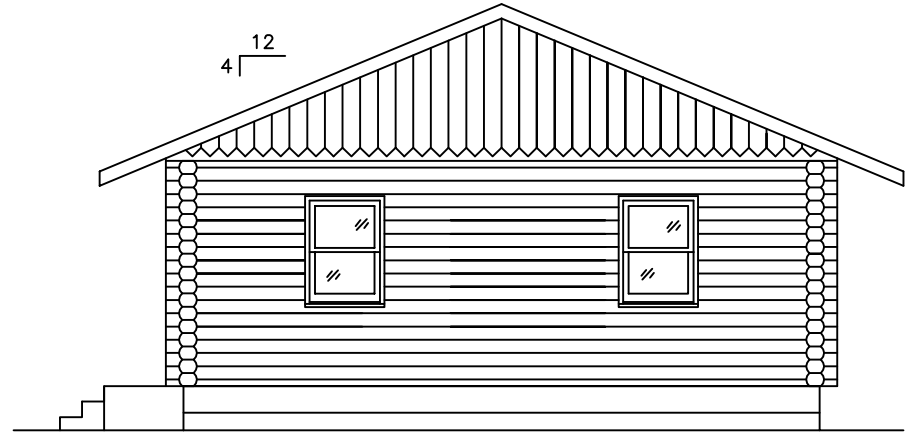
RIGHT ELEVATION
